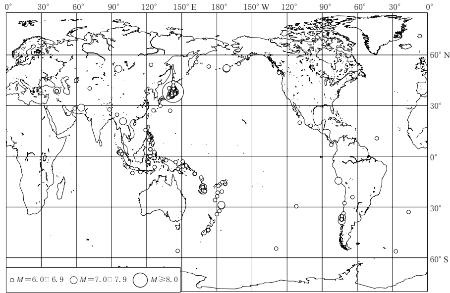
2011 年世界地震震中分布图 Epicentral distribution all over the world in 2011
