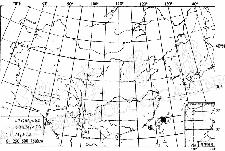
1994 年中国及邻区地震震中分布图
