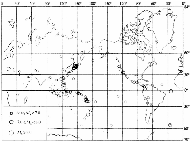
1994 年世界地震震中分布图
