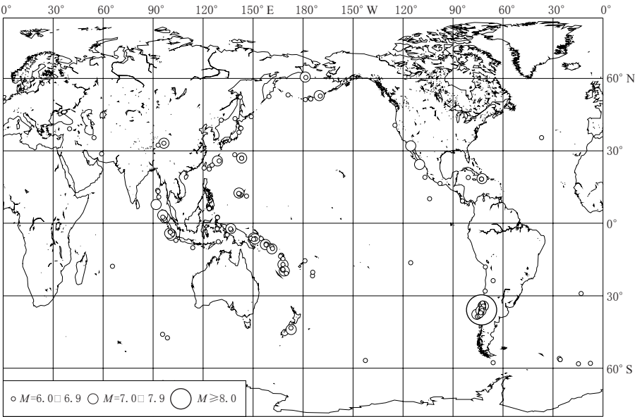
2010 年世界地震震中分布图 Epicentral distribution all over the world in 2010
