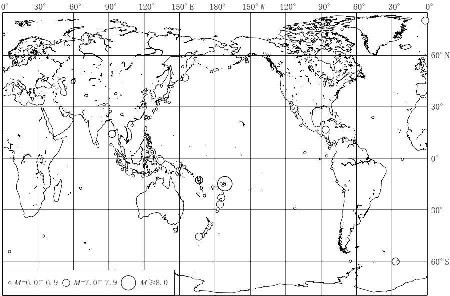
2009 年世界地震震中分布图 Epicentral distribution all over the world in 2009
