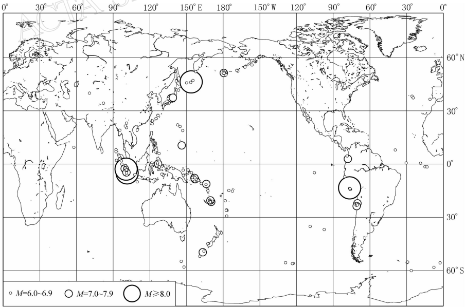
2007 年世界地震震中分布图 Epicentral distribution all over the world in 2007
